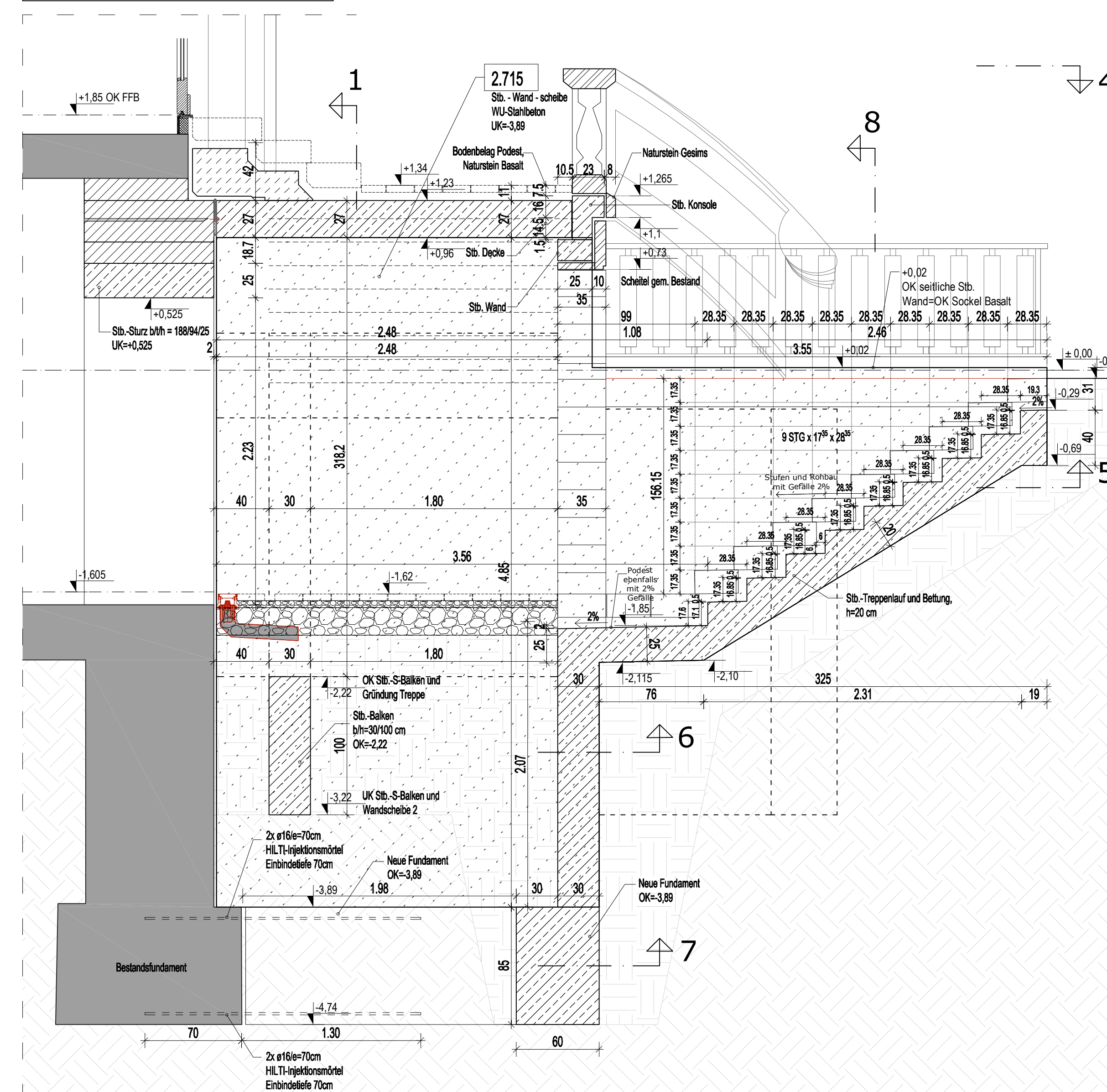
Schnitt 2-2, M. 1:25
