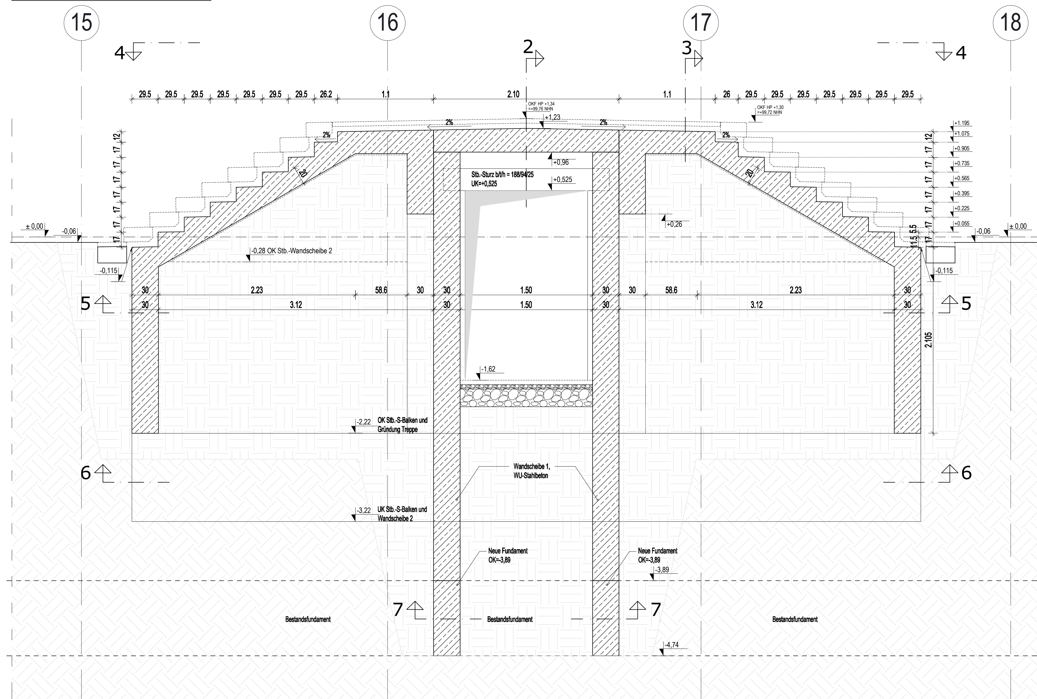
Schnitt 1-1, M. 1:25
