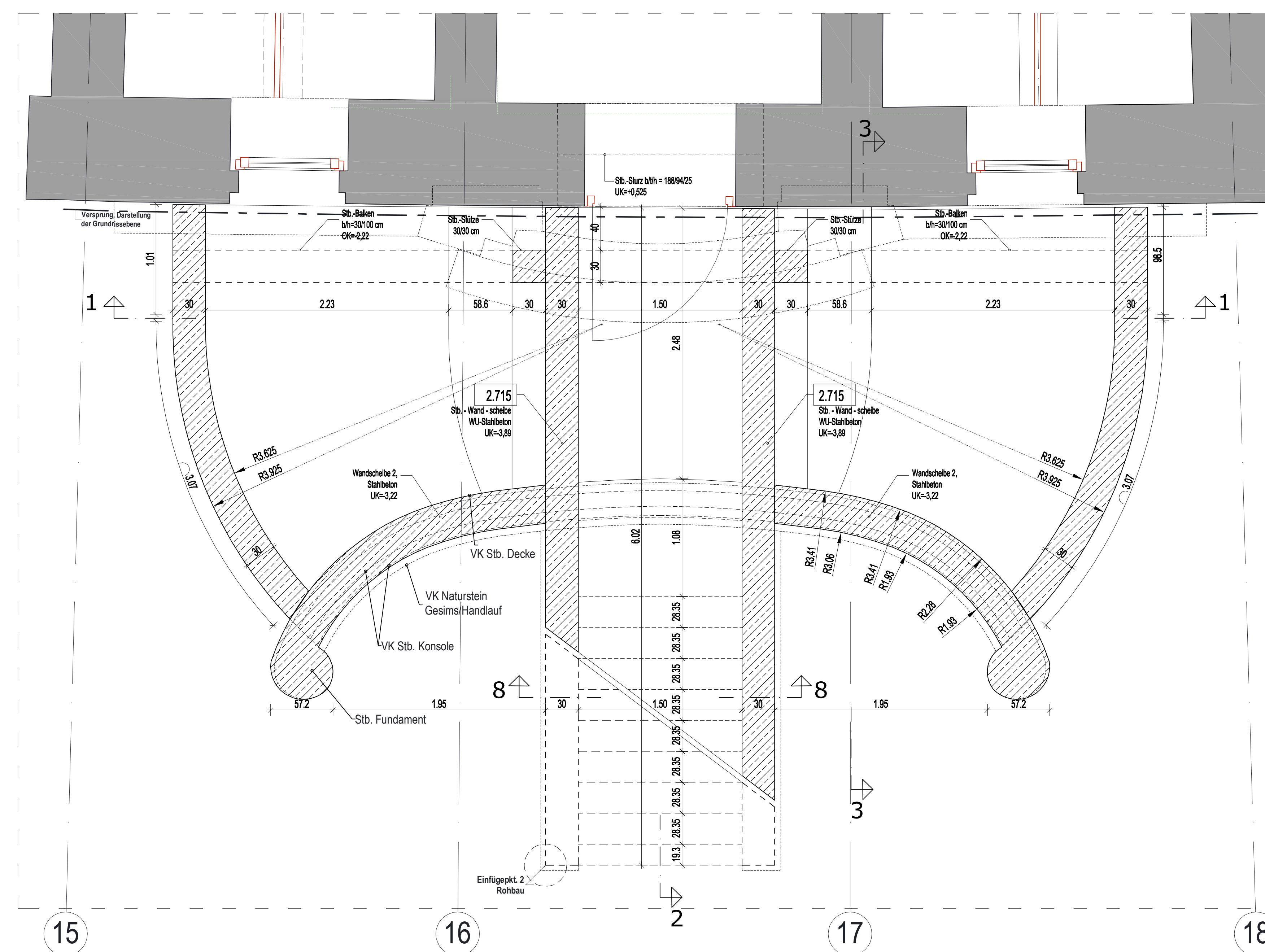
Grundrisse UG, Schnitt 5-5, M. 1:25
